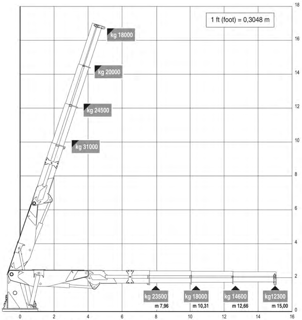
Heila 23015-3SL Crane
